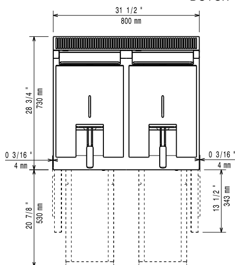
Boven aanzicht
